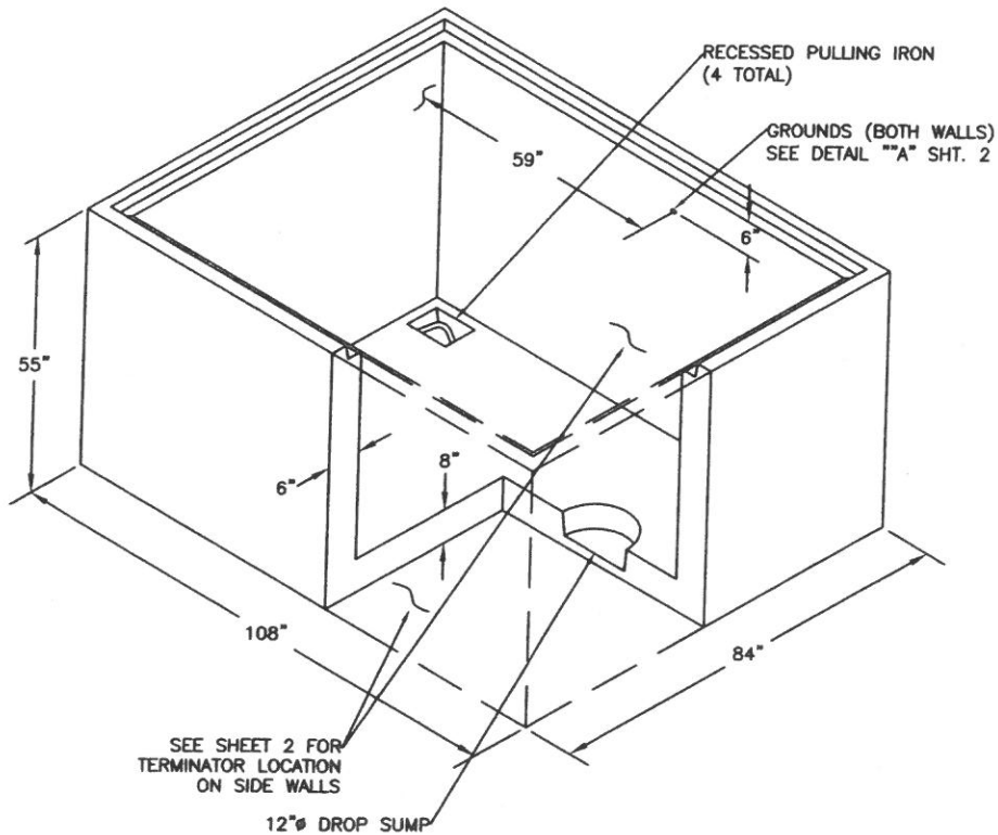
R.E.U. SWITCH VAULT
